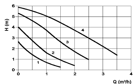
Pumpendiagramm Wilo RS 20/70r
