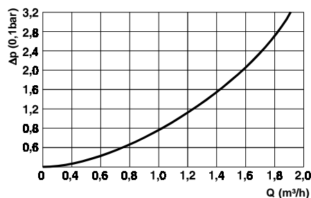
Wasserseitiger Widerstand bezogen auf \Delta t=15K
