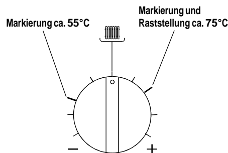
Markierungen am Heizungstemperaturregler
