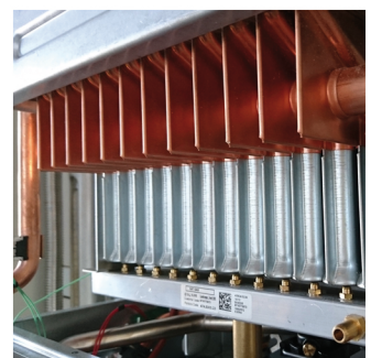
Bi-Metallbrenner
